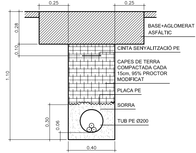
C2 (ENDESA) 1 CIRCUIT EN CALÇADA ASFALT
