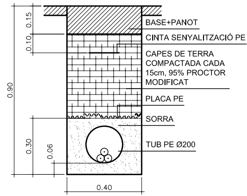
B2 (ENDESA) 1 CIRCUIT EN VORERA
