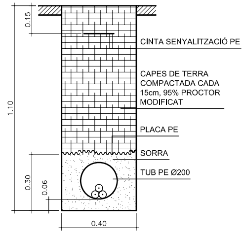
A2 (ENDESA) 1 CIRCUIT EN TERRA
