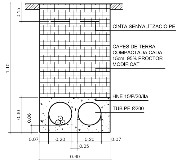
H2 (ENDESA) SORTIDA SUBESTACIÓ 1C EN TERRA+2TF EXECUCIÓ PER PART D'ENDESA
