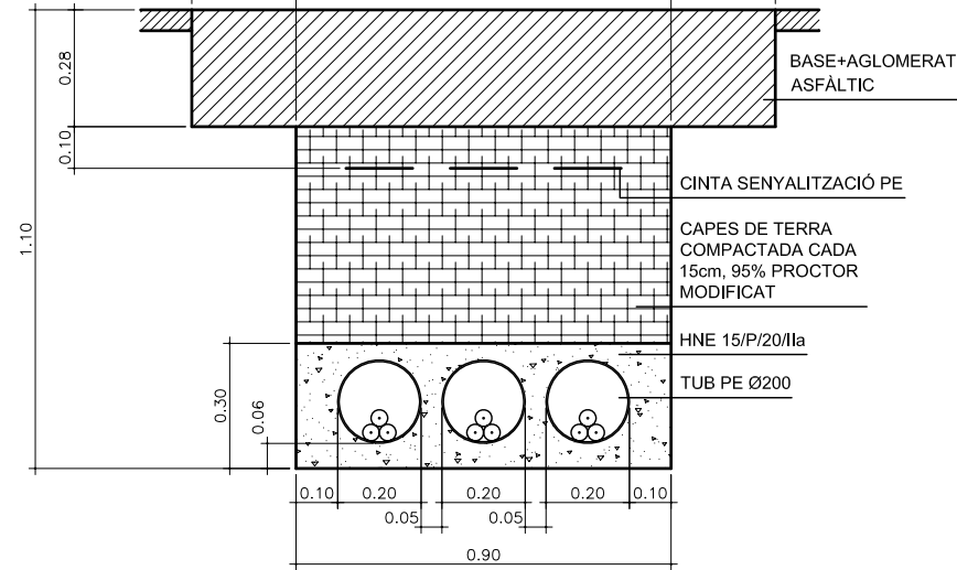
H2 (ENDESA) SORTIDA SUBESTACIÓ 1C EN TERRA+2TF EXECUCIÓ PER PART D'ENDESA
