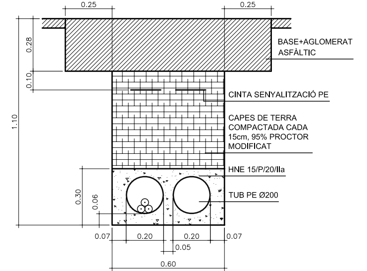
D2 (ENDESA) ENCREUAMENT 1C+2TF
