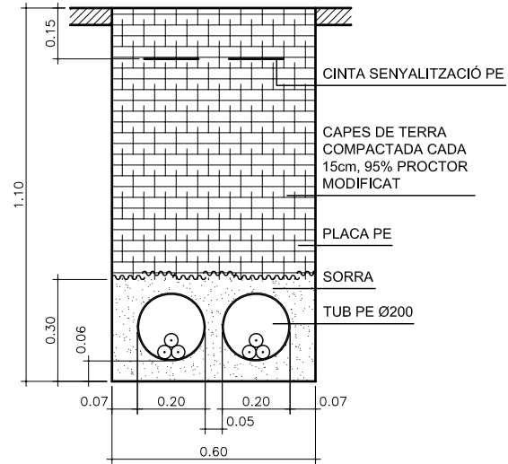
E2 (ENDESA) 2 CIRCUITS EN TERRA
